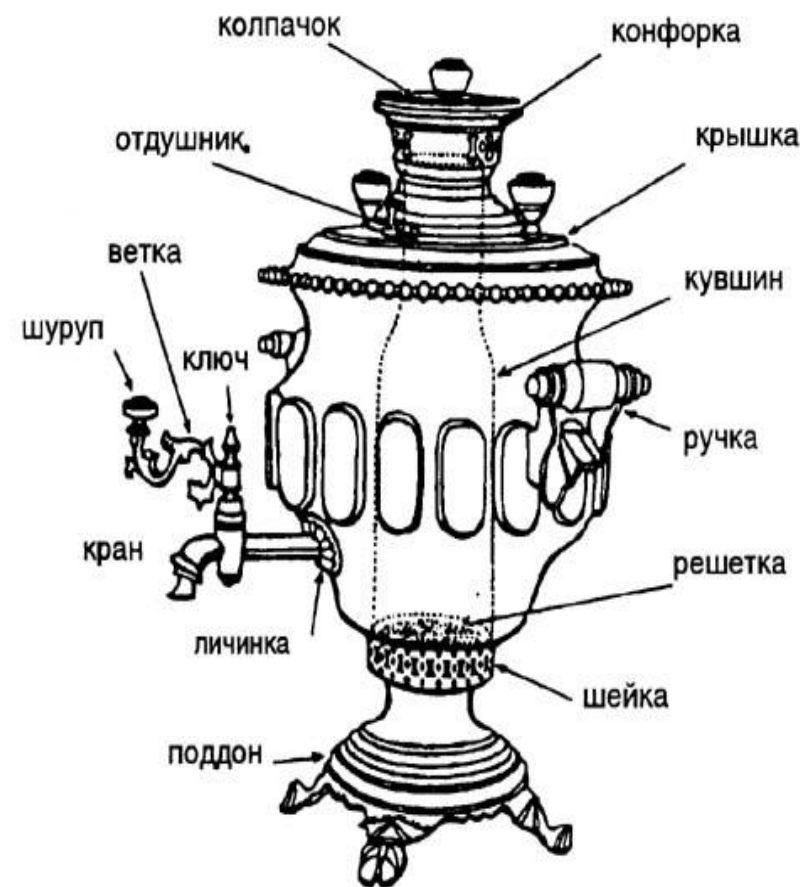
Схема устройства самовара
